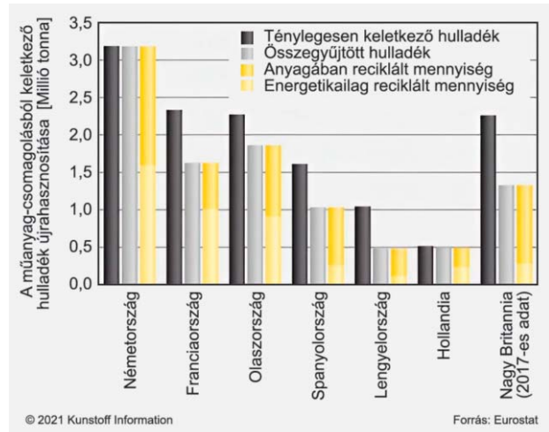
1. ábra. A műanyag-csomagolásból keletkező hulladék újrahasznosítása a duális rendszer szerint regisztrált és a reciklási technológiai adatok alapján az EU 7 tagállamában.
