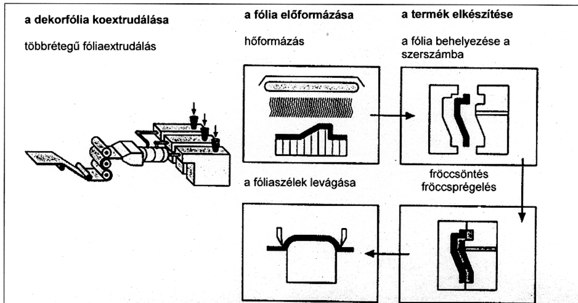
3. ábra Műanyag karosszériaelemek előállítás a PMF technológia segítségével
