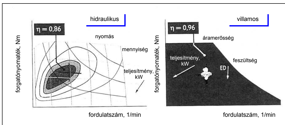
1. ábra A feldolgozási ablak (sötét terület) hidraulikusan (bal oldali kép) és villamosan hajtott adagolórendszerrel (jobb oldali kép)
