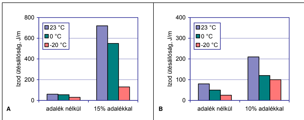
4. ábra PBT hornyolt próbatestenen mért Izod ütésállósága Elvaloy PT862 adalékkal és anélkül. (A: erősítetlen típus, B: 30% üvegszállal erősített típus.)
