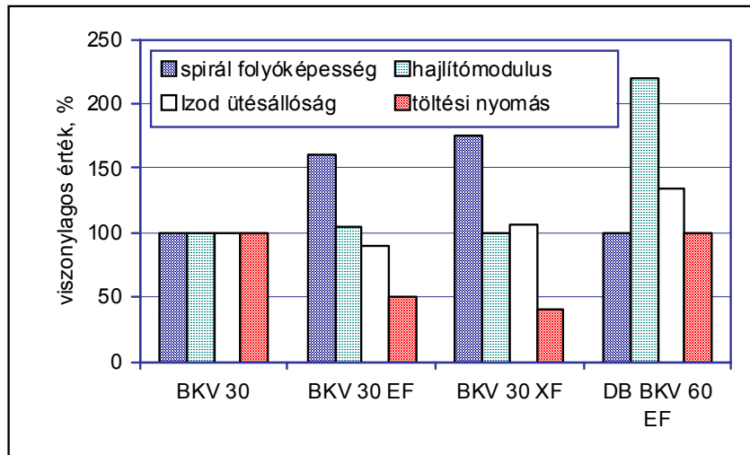
1. ábra A nagy folyóképességű, különböző üvegszáltartalmú BKV EF és XF poliamidok standard BKV 30-éhoz viszonyított tulajdonságai
