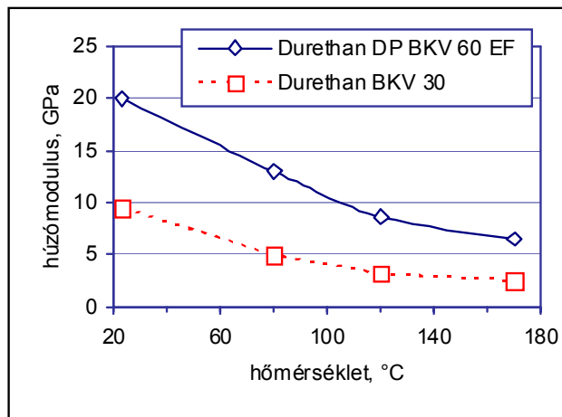
2. ábra A 60% üvegszálat tartalmazó nagy folyóképességű és a 30% üvegszálat tartalmazó standard BKV húzómodulusának változása a hőmérséklet hatására
