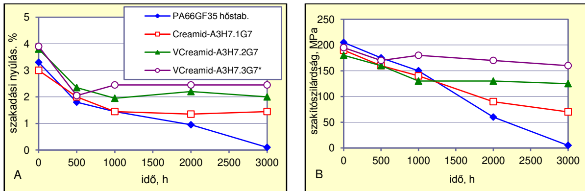
2. ábra Egy 35% üvegszál tartalmú hőstabilizált, de térhálósítás nélküli PA66, továbbá egy hőstabilizált de nem térhálósított Creamid és két hőstabilizált és sugárzással térhálósított V-Creamid szakadási nyúlásának (A ábra) és szakítási szilárdságának (B ábra) változása az idő függvényében 220 °C-on végzett hőöregítés alatt. A *-gal jelölt V-Creamidnál a Shield -technológiát alkalmazták
