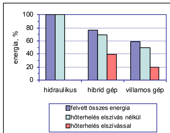
2. ábra Különböző módon hajtott fröccsgépek tisztatérrel terhelő hőenergiája
