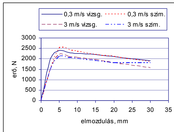
2. ábra Egy PA/ABS próbatest gyors szakítási vizsgálatának mért (vizsg.) és számított (szim.) görbéi
