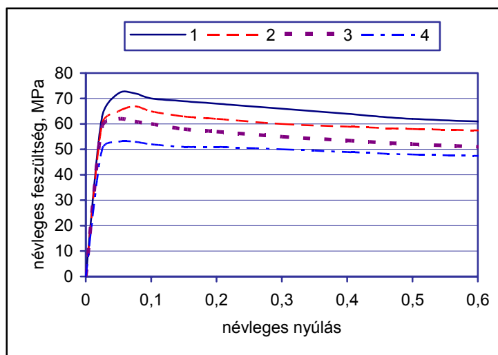
4/b ábra PA6 minták névleges feszültség-nyúlás görbék különböző nyújtási sebességek mellett: 1. 10^2 /s, 2. 10^1 /s, 3. 10^0 /s, 4. 10^{-1} /s
