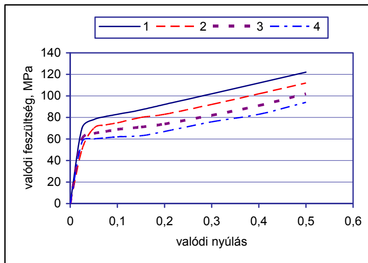
4/a ábra PA6 mintákon mért valódi feszültség-nyúlás görbék különböző nyújtási sebességeken: 1. 10^2 /s, 2. 10^1 /s, 3. 10^0 /s, 4. 10^{-1} /s
