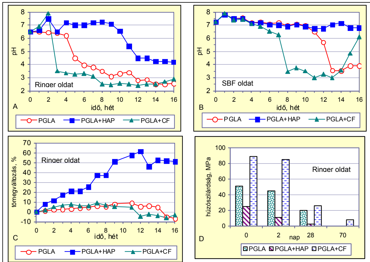
4. ábra A fiziológiás (Ringer) oldat (A kép) és a szimulált testfolyadék (SBF oldat) (B kép) pH-jának változása az idő függvényében a bennük inkubált próbatestek hatására; továbbá a Ringer oldatban kezelt próbatestek tömegének (C kép) és húzószilárdságának (D kép) változása az inkubálás időtartamának függvényében
