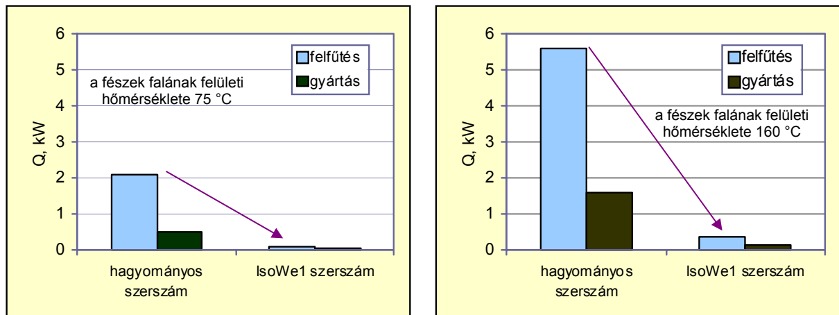
2. ábra Egy hagyományos és egy IsoWE szerszám energiafelvétele felfűtéskor és gyártás közben 75 °C-ra, ill. 160 °C-ra temperált szerszámban
