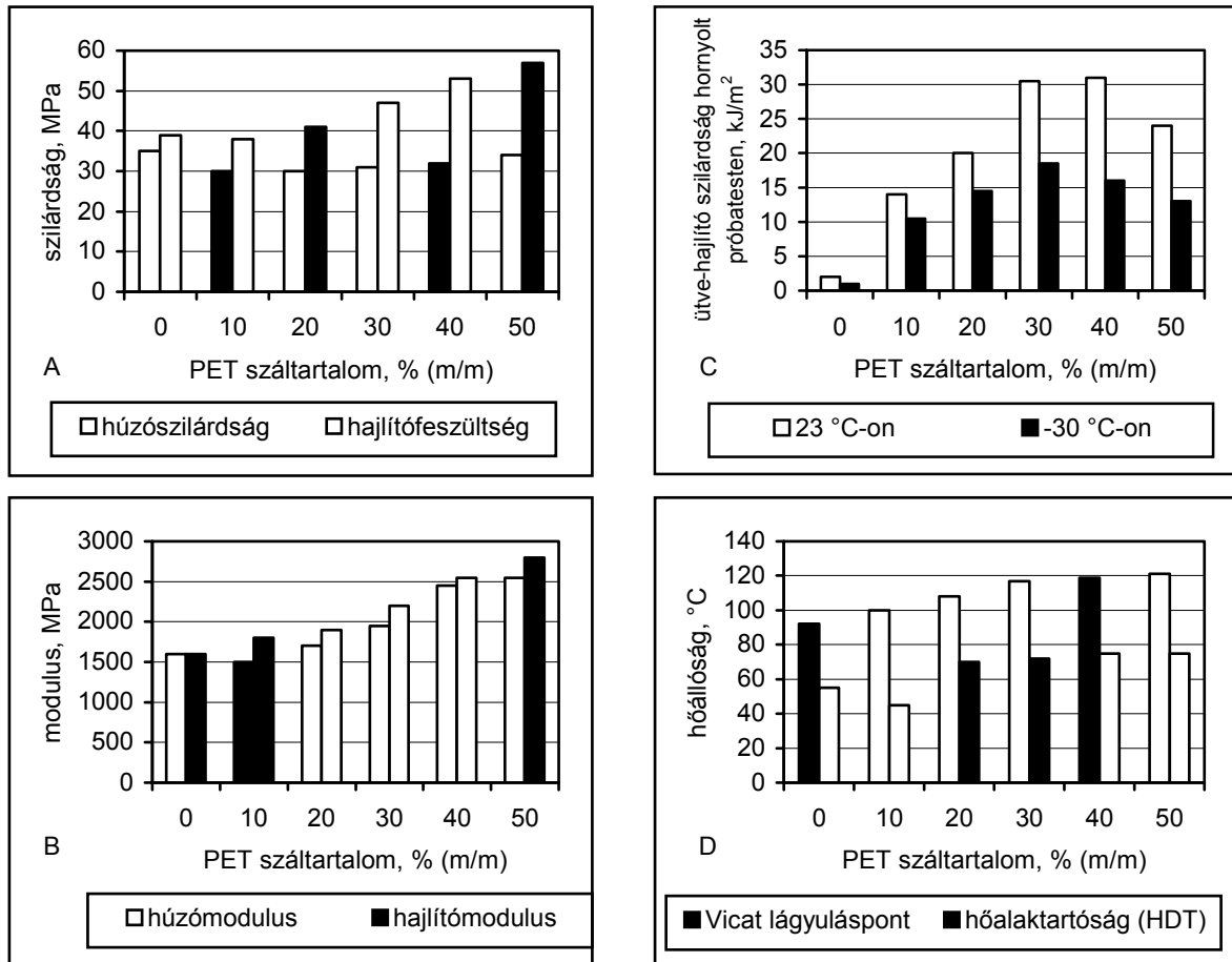
5. ábra PET szál tartalmazó PP keverékek tulajdonságai a száltartalom függvényében
