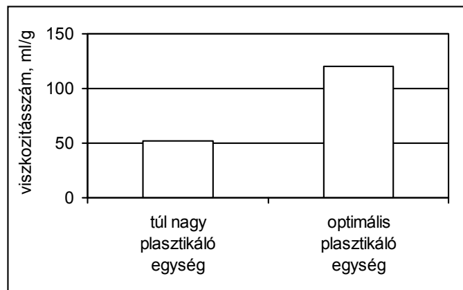
3. ábra A plastikáló egység hatása a 10% őrleményt tartalmazó Ultramid B3UG4 típusú PA 6 viszkózitásszámára
