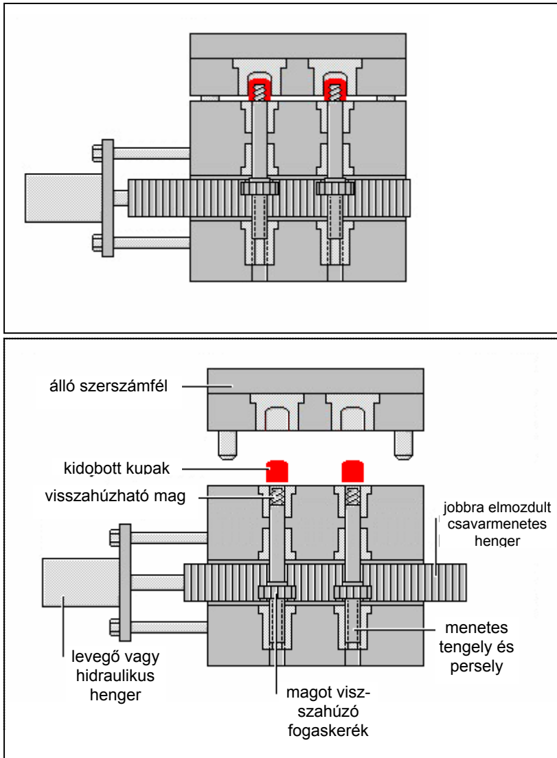
1. ábra Belső csavarmentes kupakok kidobása a kétfészkes szerszámából csavarmentes henger és fogaskerékkel visszahúzzható magok segítségével (unsrewing tool)
