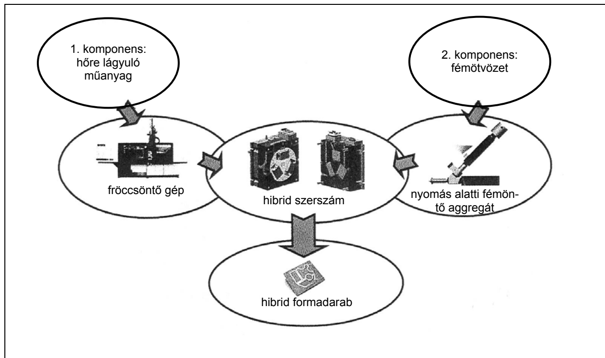
1. ábra A műanyagból és a fémolvadékból gyártott hibrid formadarab gyártósorának vázlatja
