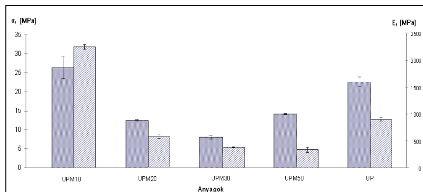
3. ábra A vizsgált anyagok hajlítószilárdsága és hajlító modulusa
