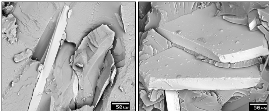
5. ábra Az 50 %(m/m) mágnesport tartalmazó roncsolt próbatetek törésfelületéről készült SEM felvételek
