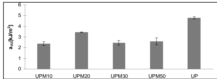
4. ábra A vizsgált minták fajlagos törési energiái
