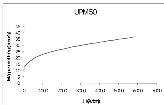
1. ábra Az 50 %(m/m) mágnesport tartalmazó minta hiszterézis görbéjének kezdő szakasza
