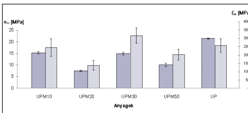
2. ábra A vizsgált anyagok szakítószilárdsága és rugalmassági modulusa
