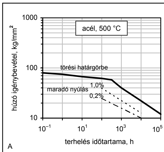
1. ábra Acél (A kép, 500 °C) és polietilén (B kép, 20 °C) tartós terhelési görbéi
