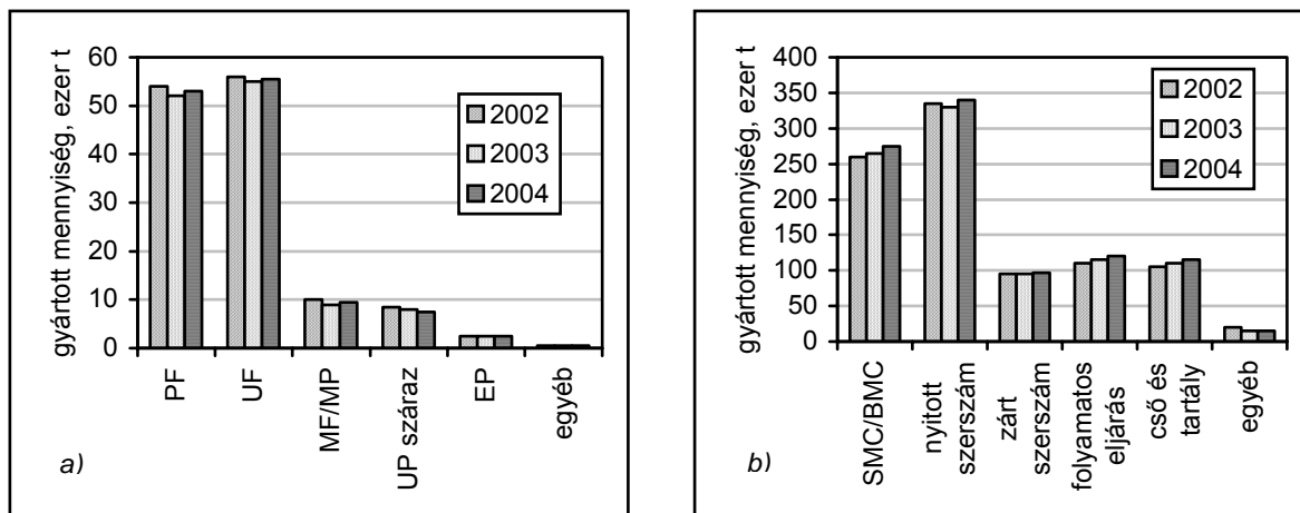
1. ábra Az Európában gyártott hőre keményedő sajtolóanyagok mennyisége 2002–2004-ben. a) kép: klasszikus sajtolóanyagok; b) kép: üvegszálás sajtolóanyagok a feldolgozási eljárás szerinti megosztásban
