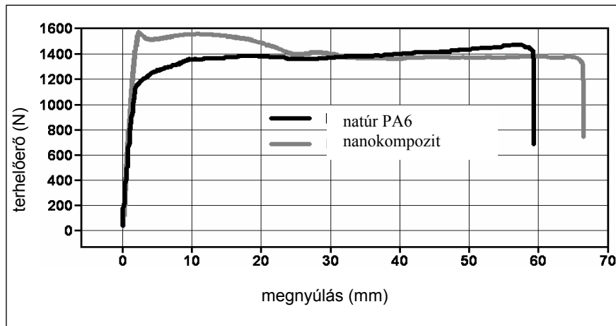
2. ábra Szakítódíagram
