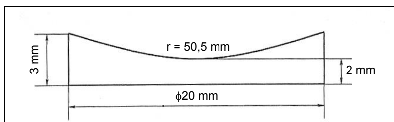
5. ábra A plán-konkáv lencse méretei
